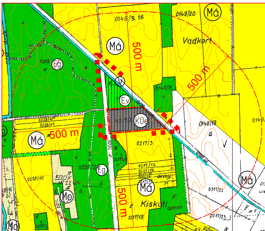
3./ Biogáz üzem területi jelölése SZK-M1c
